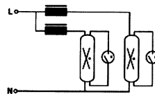
Рис. 3. Схемы электрические некомпенсированные (выполняются по заказу потребителя)
