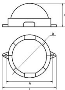
Рис. 1. Общий вид светильника DBV 06-01
