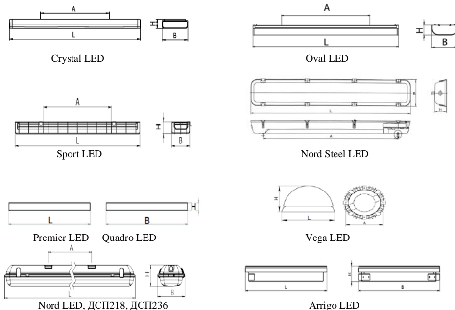
Рис. 1. Общий вид и расположение точек крепления (размер А)
