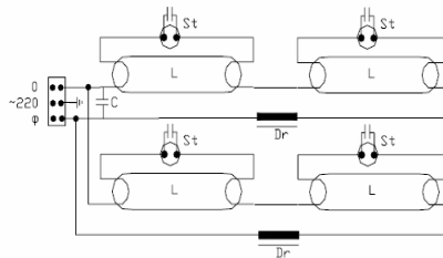
Рис. 2. Схема включения светильников с ЭМПРА
